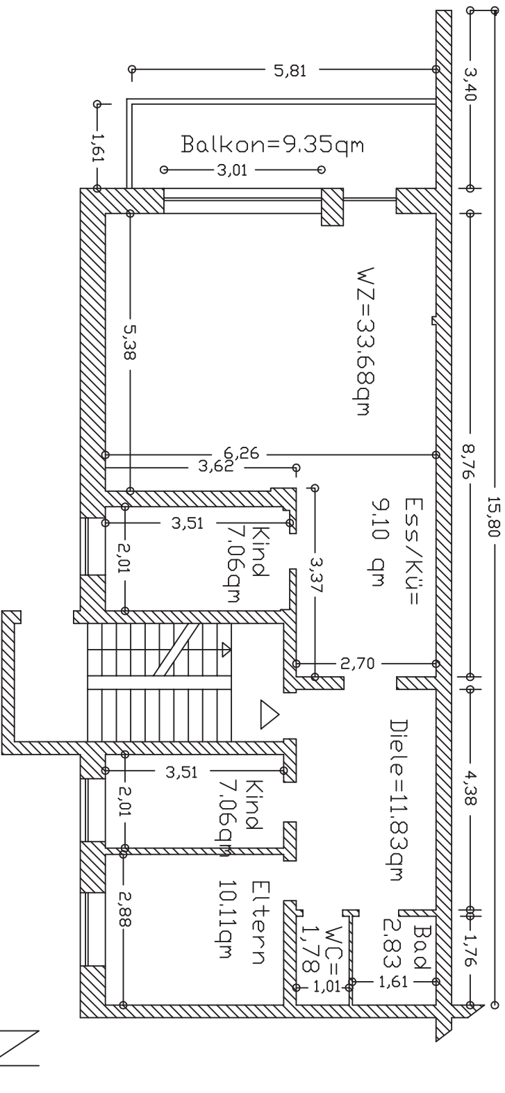
Erdgeschoss, Dorfstrasse 11, Garbsen Maßstab 1:100
